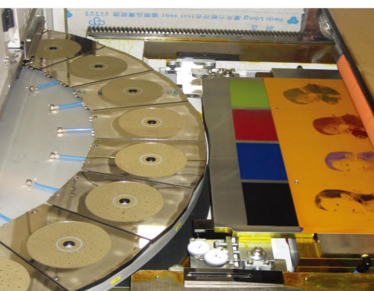
印刷圓盤及真空吸版裝置
