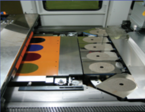
印刷輸送帶及真空吸版裝置
