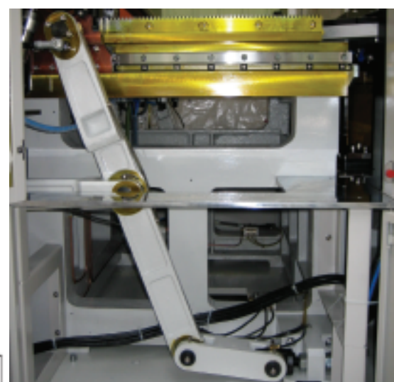
機械手臂
